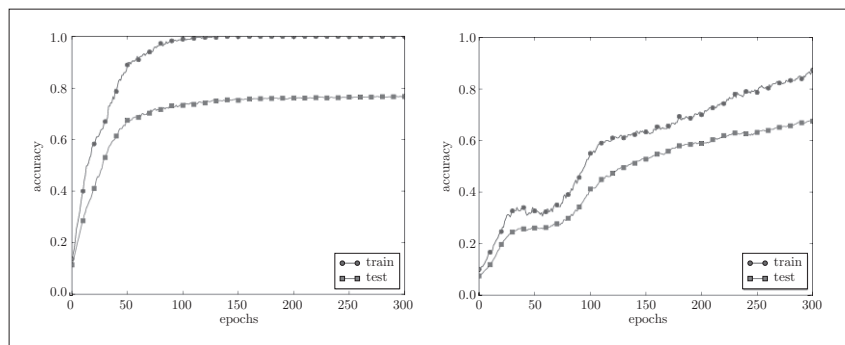
图6-23 左边没有使用Dropout,右边使用了Dropout(dropout_rate=0.15)
