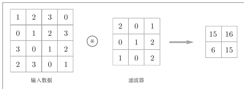
图 7-3 卷积运算的例子：用“ \circledast ”符号表示卷积运算
